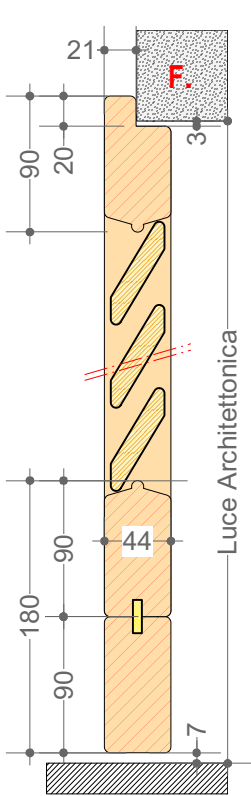
F. senza traverso centrale
