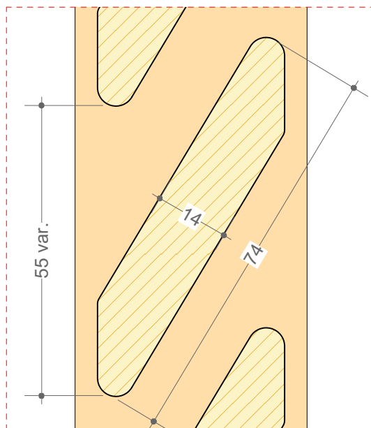
F. senza traverso centrale
